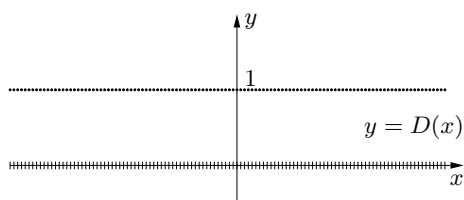
Rys. 1.38. Wykres funkcji Dirichleta
