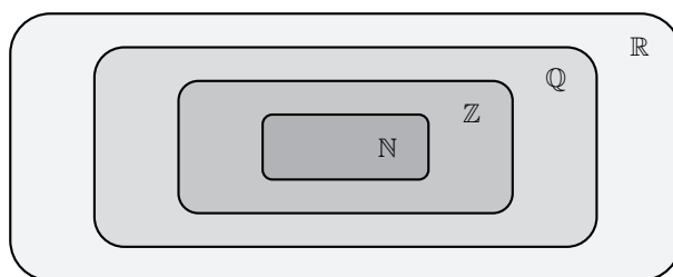
Rys. 1.1. Relacje \mathbb{N} \subset \mathbb{Z} \subset \mathbb{Q} \subset \mathbb{R}
