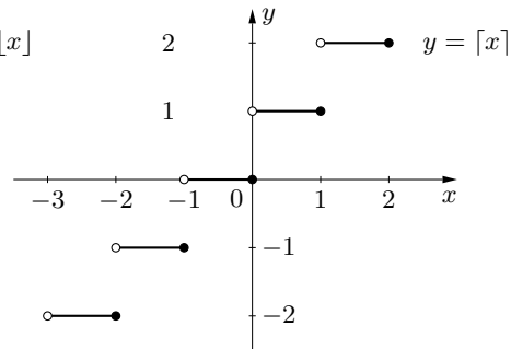
Rys. 1.35. Wykres funkcji sufit
