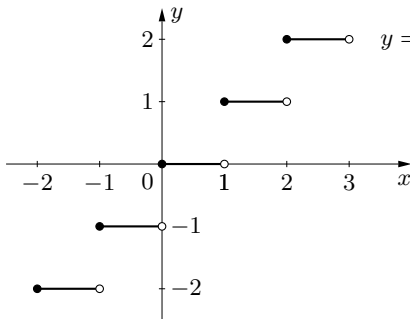
Rys. 1.34. Wykres funkcji podłoga
