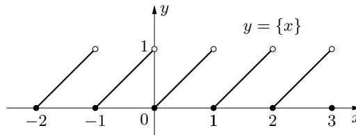
Rys. 1.36. Wykres funkcji część ułamkowa
