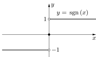
Rys. 1.37. Wykres funkcji signum
